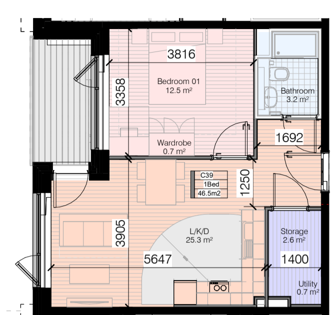
Apt Type 1 Bed (D)-2nd-6th Floor 1 : 100
